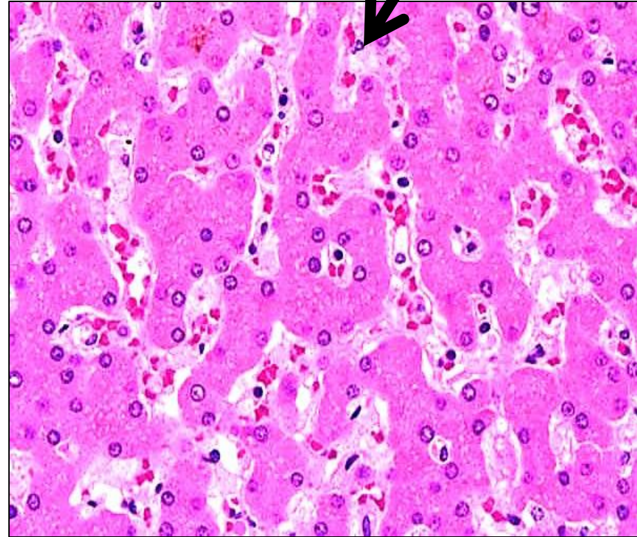
sinusoids
