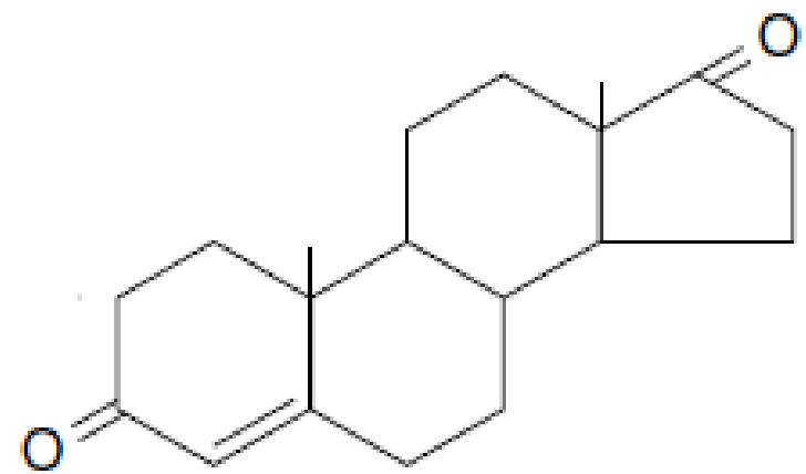
Androstenedione
