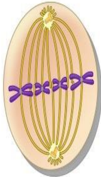
Metaphase
