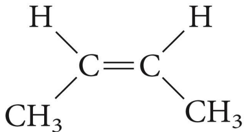
cis-2-butene
