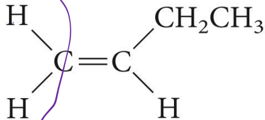
1-butene
