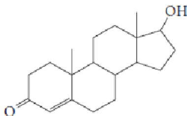
testosterone (testes) mp 155°C
