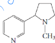
nicotine bp 246°C
